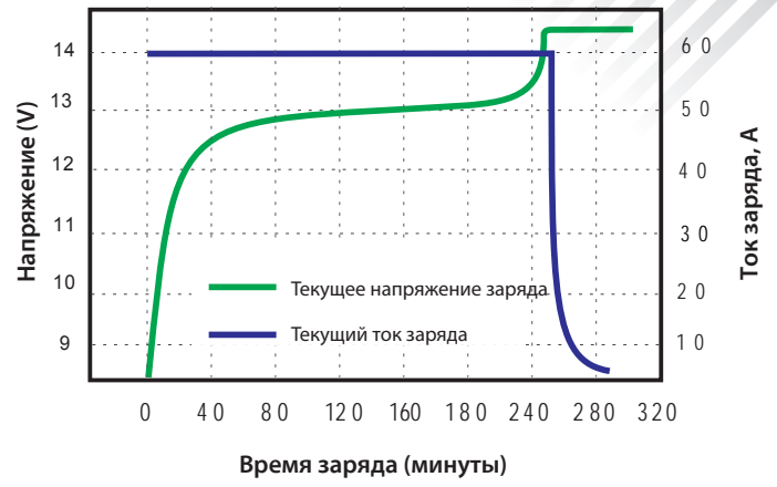
Характеристики заряда при 0.5C 25°C
