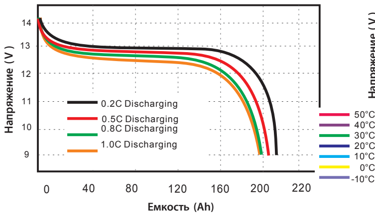
Графики разряда разными токами при 25°C
